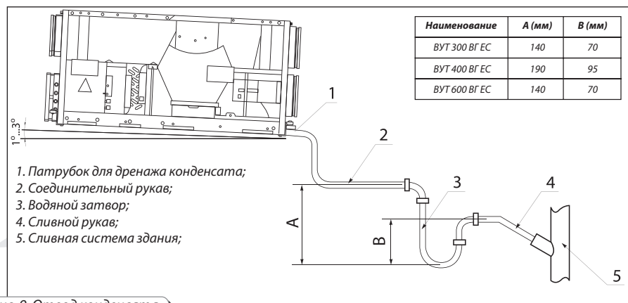
Рис. 9. Отвод конденсата
