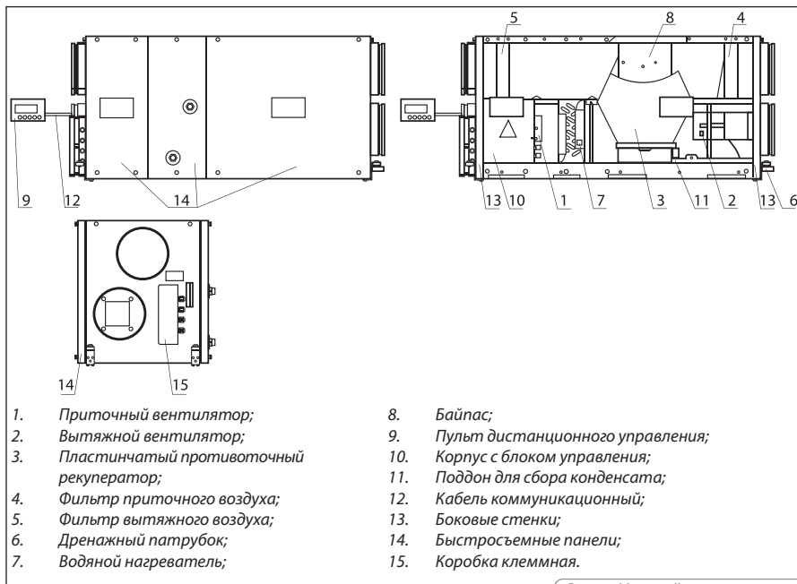
Рис. 4. Устройство установки
