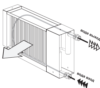
Рис. 7. Подключение водяного нагревателя
