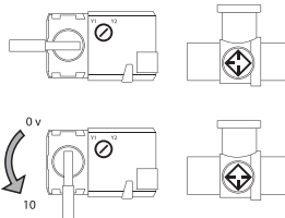
Сервопривод трехходового вентиля
