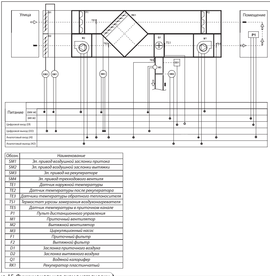
Рис. 15. Функциональная схема установки
