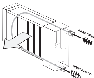
а) Прямоточное подключение
