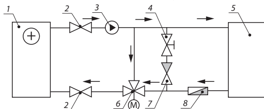
Схема смесительного узла
